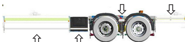
RESTS-W: Tiras reflectoras brancas montadas na parte lateral do chassis (protecção inferior/caixa de ferramentas/entre os guarda-lamas/saliência traseira).
