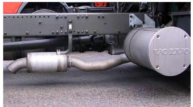
Silenciador horizontal com saída para a retaguarda.
