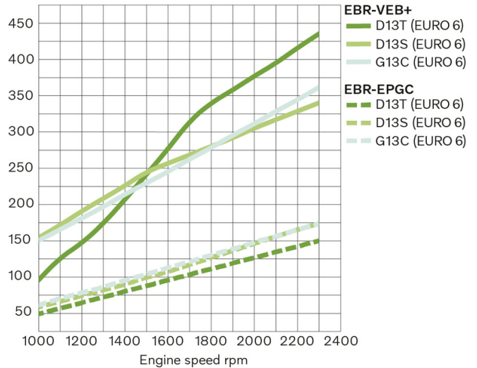
D13 engines Euro 6
