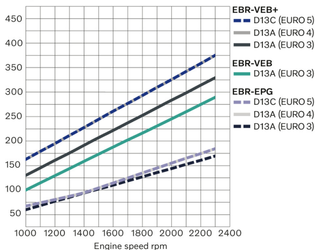
D13 engines EURO 3-5
