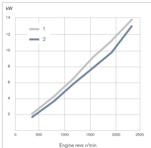
Consumo de energia a 12,5 bar. 1: Embraiagem dupla; 2: Sem embraiagem.
